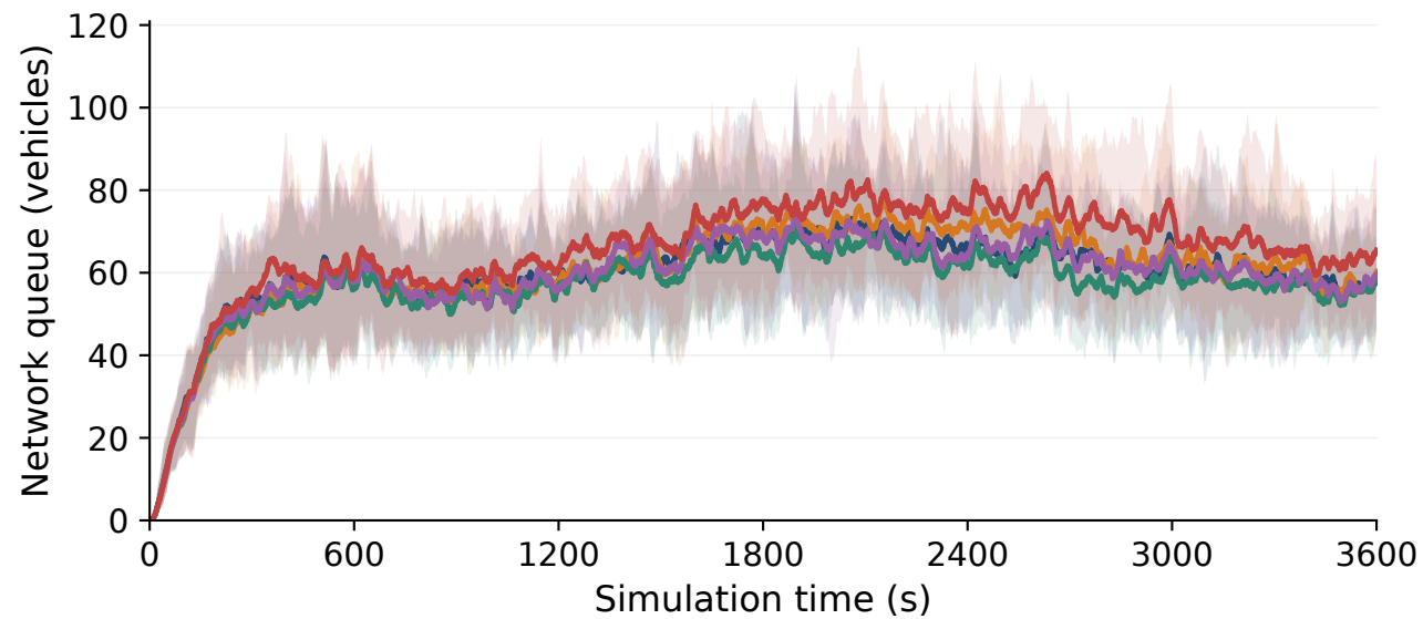
IQLL
